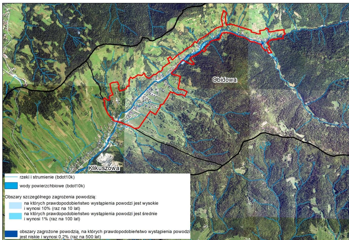
Ryc. 13. Obszary szczególnego zagrożenia powodzią
