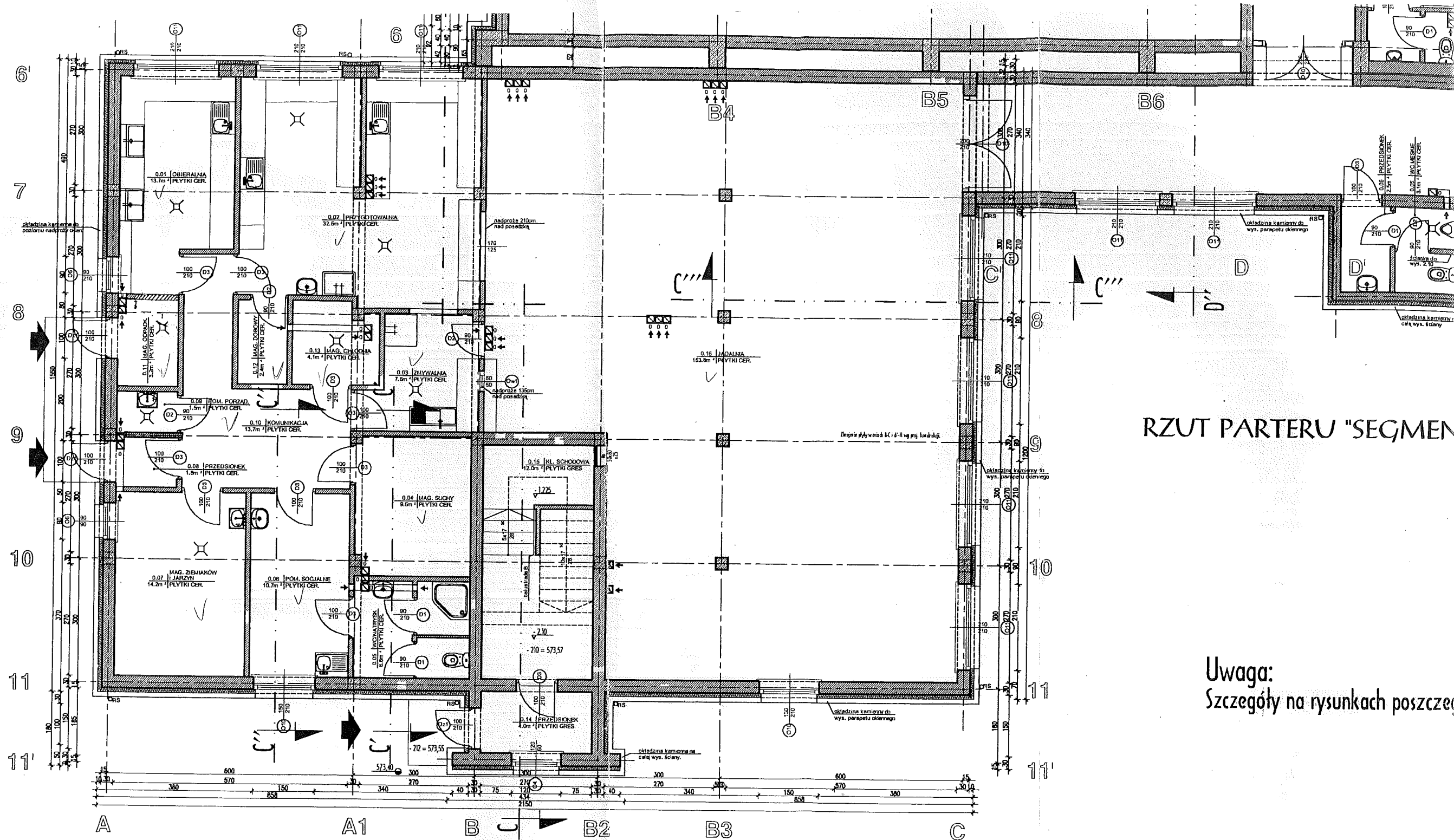
RZUT PARTERU "SEGMENT C" SKALA 1:100
